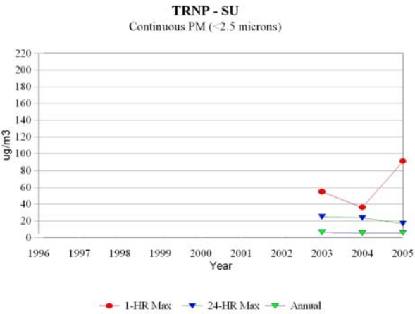
Figure A4-12 TRNP - NU(cont.)/TRNP - SU Trends
